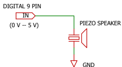
(d) Piezo speaker without resistor
